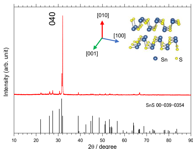
XRD分析結果
