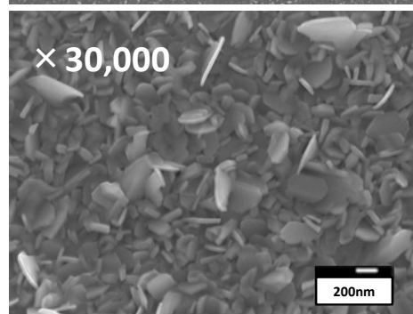
SEM観察画像
